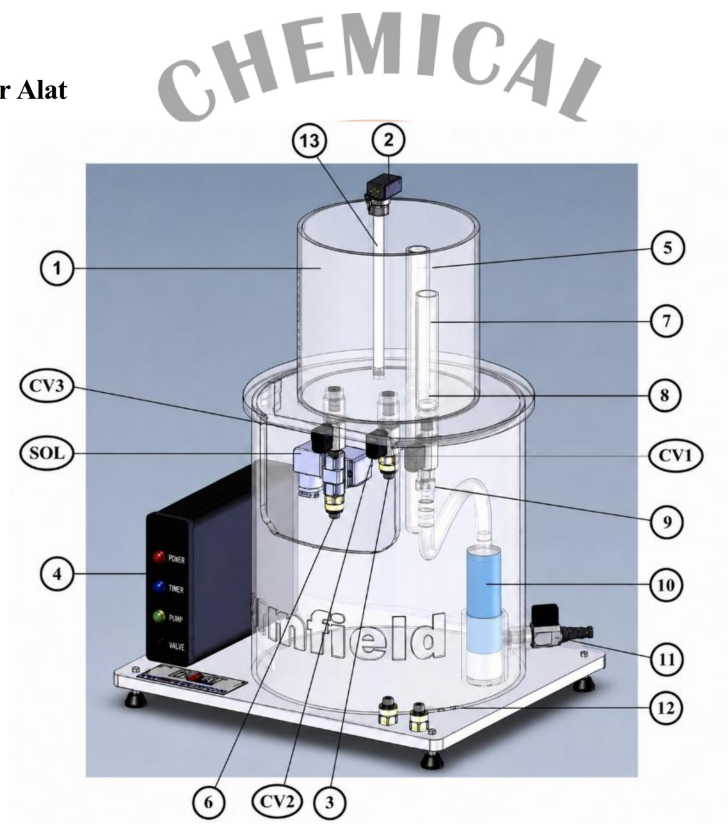
Gambar 3.2 Alat PCT 50 level control dan bagian-bagiannya
